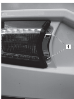
Bild 202: Demontera baklampan
