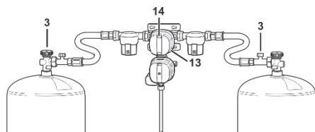
Bild 115: Gastryckregulatorsats
