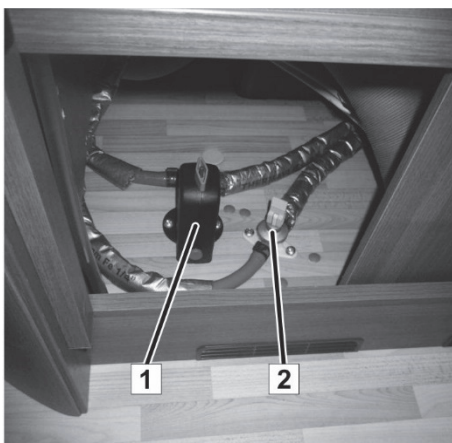
Bild 105: Avtappningsventiler för värmeaggregatet TRUMA Combi
