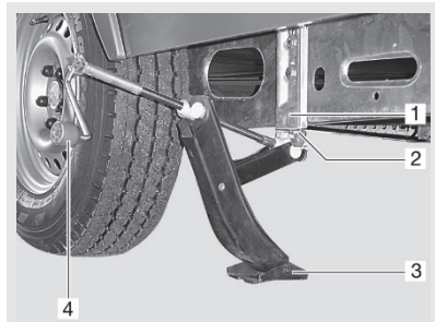
Bild 199: Domkraft AL-KO
