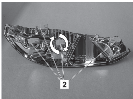
Bild 203: Baklampa (baksida)
