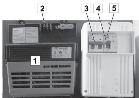
Bild 60: Omformare (nätadapter) (1) och automatsäkringar
