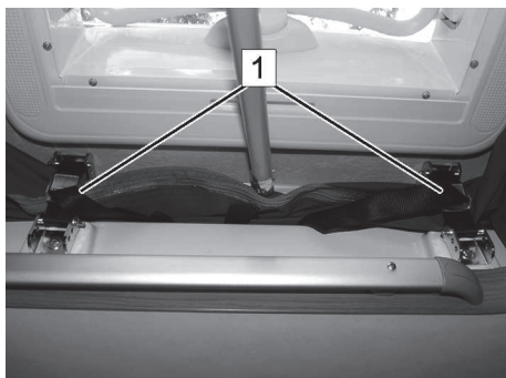
Bild 169: Taklås (1)
