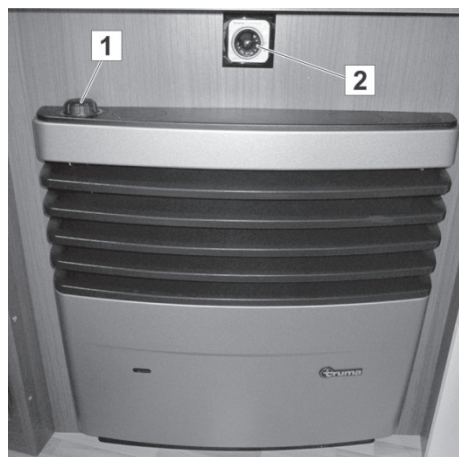
Bild 125: TRUMA-värmeaggregat
