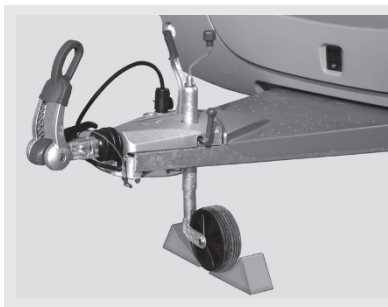
Bild 196: Säkra stöd hjulet
