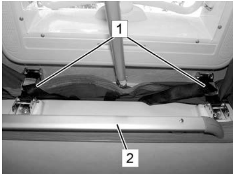
Afb. 169: Hefdak uitklappen
