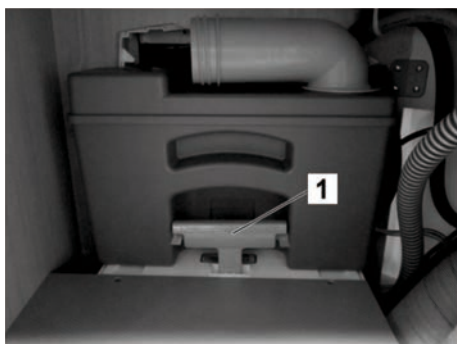
Afb. 179: Fecaliëntank in het afvalkanaal
