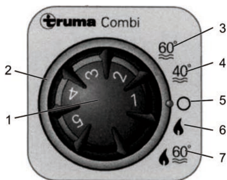
Afb. 120: TRUMA-regelunit voor verwarming en warmwater
