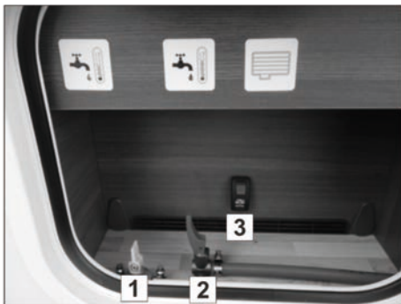
Afb. 95: Aftapkleppen ALDE
