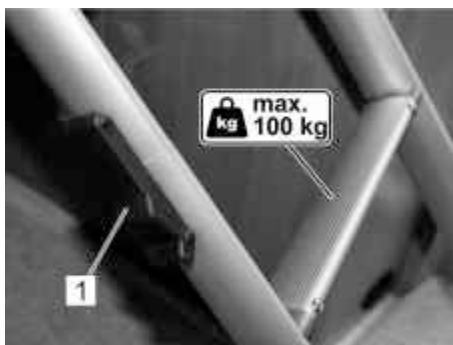
Afb. 170: Vergrendeling (1) van de klimladder
