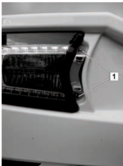
Afb. 201: Achterlicht weer aanbrengen
