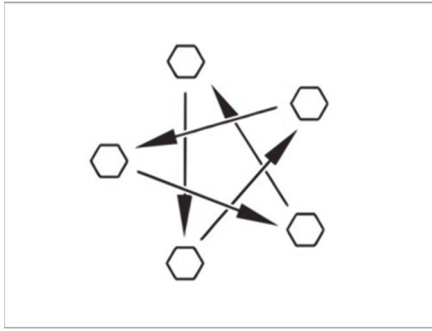
Abb. 195: Radmuttern oder Radschrauben über Kreuz anziehen
