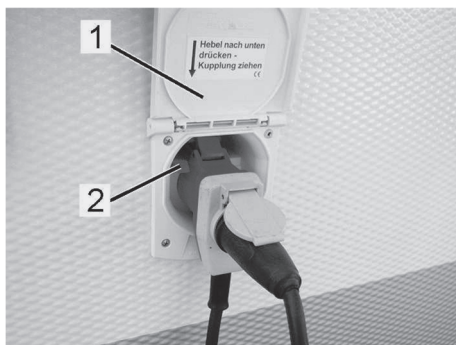
Abb. 100: Netzanschluss
