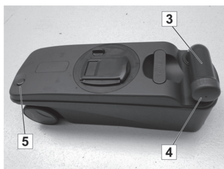
Abb. 173: Fäkalientank entleeren
