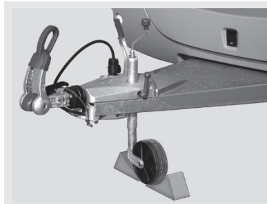
Abb. 196: Stützrad sichern
