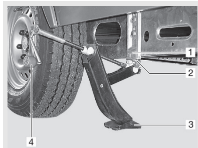
Abb. 199: Wagenheber AL-KO
