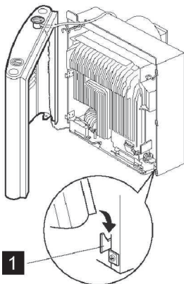
Abb. 129: Heizverkleidung aufgeschwenkt
