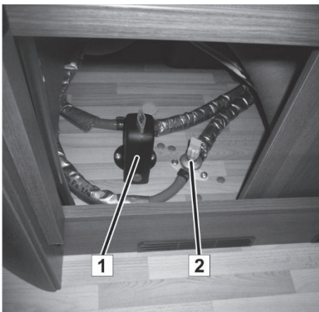
Abb. 105: Ablasventile TRUMA-Combi-Heizung
