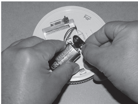
Abb. 206: Blockbatterie austauschen
