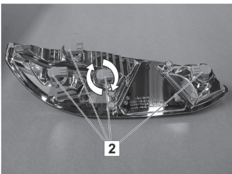
Abb. 203: Heckleuchte (Rückseite)
