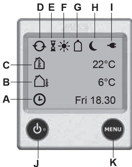
Abb. 136: Bedienelemente
