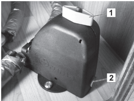
Abb. 106: Sicherheits-Ablassventil offen
