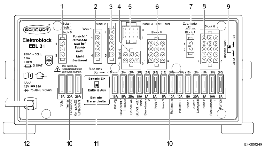
Bild 66 Elektroblok (EBL 31)
