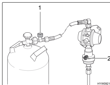
Bild 7 Gasregler (MonoControl)
