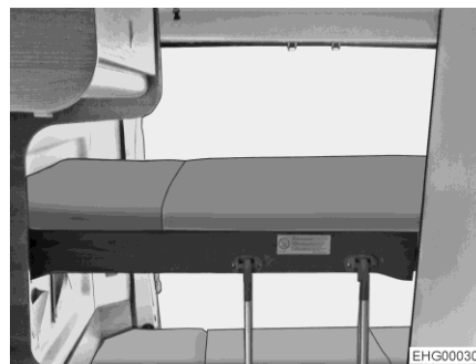
Kuva 42 Kerrossänky ja paikalleen ripustetut tikkaat
