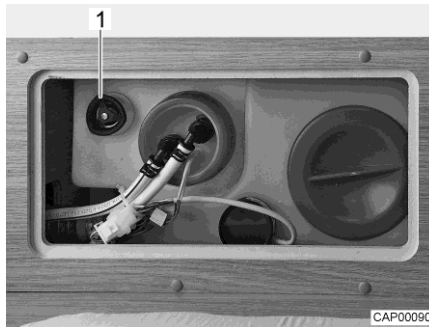
Kuva 96 Vesisäiliö kääntökahvalla
