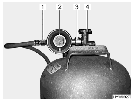
Kuva 63 Kaasupullon liitântä
