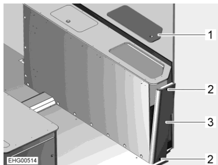
Kuva 109 Oikeanpuoleinen vuodelaatikko
