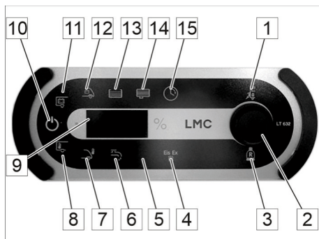
Fig. 58: Pannello di comando e controllo LT 632
