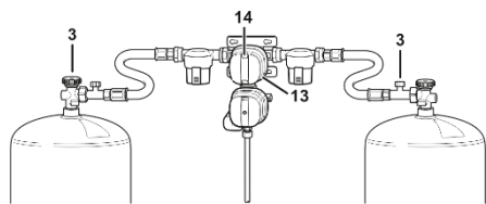
Fig. 108: Set regolatore di pressione del gas
