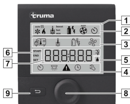
Fig. 120: Unità di comando digitale TRUMA CP Plus
