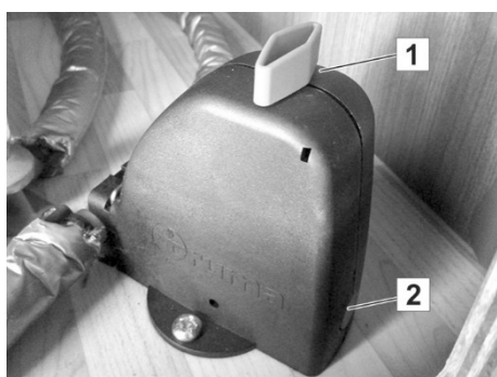
Fig. 157: Valvola di scarico di sicurezza chiusa
