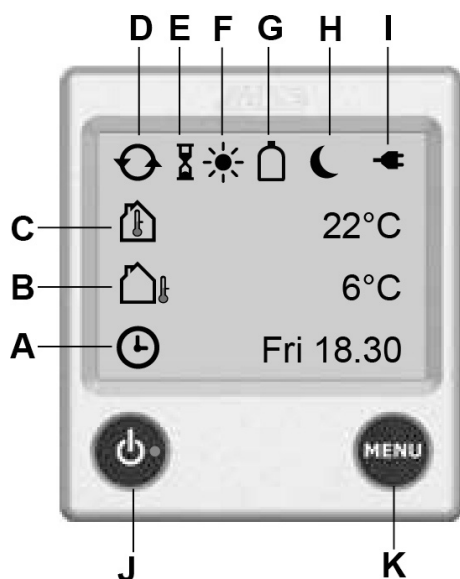
Fig. 80: Elementi di comando
