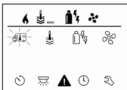
Fig. 123: Display livello di impostazione
