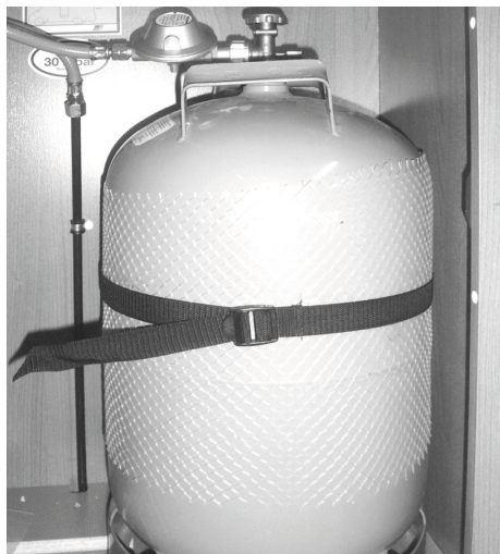
Fig. 103: Portagas
