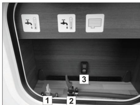
Fig. 93: Valvole di scarico ALDE
