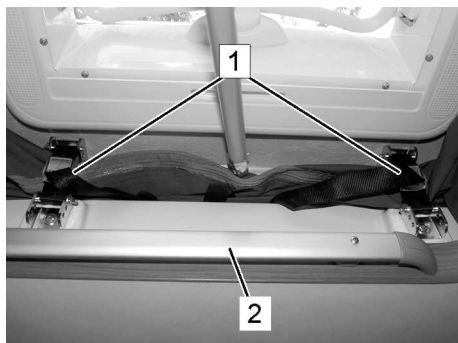
Fig. 173: Aprire il tetto sollevabile ribaltandolo
