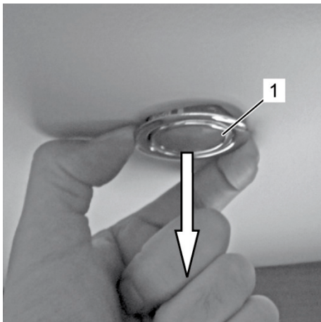
Fig. 199: Estrarre il LED
