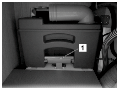
Fig. 182: Serbatoio acque nere nel vano WC
