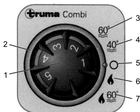
Fig. 118: Unità di comando TRUMA per riscaldamento e la preparazione di acqua calda
