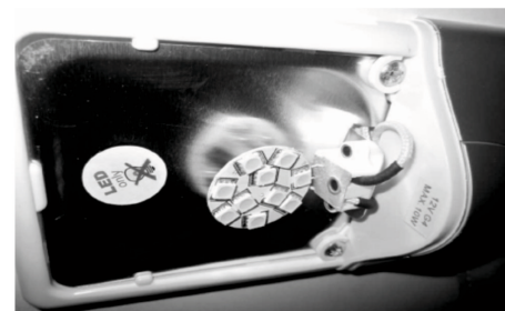
Fig. 153: Inserimento corpo illuminante a LED
