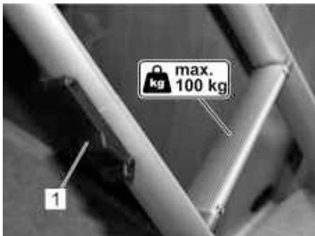
Fig. 130: Meccanismo di bloccaggio (1) della scaletta
