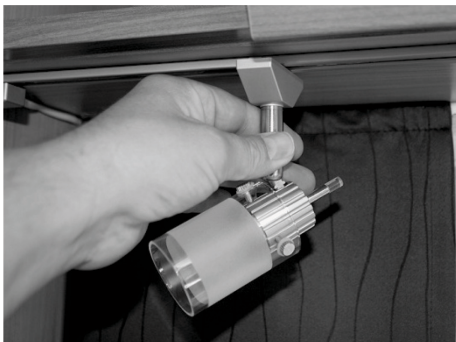
Fig. 135: Spostamento faretto LED
