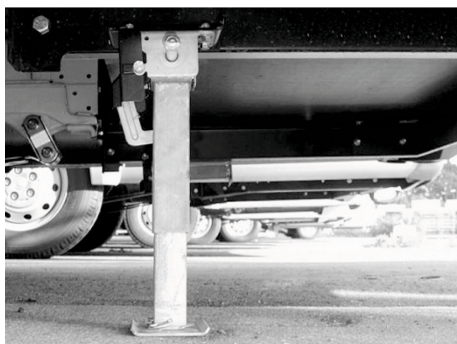
Fig. 13: Piedino di stazionamento posteriore fuoriuscito
