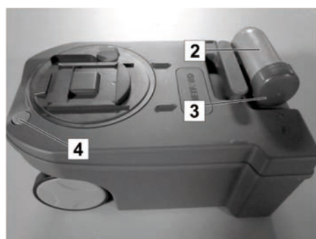
Fig. 196: Svuotare il serbatoio acque nere
