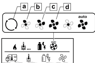
Fig. 140: Simbolo velocità del ventilatore
