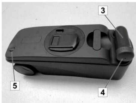
Fig. 193: Svuotare il serbatoio acque nere
