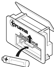
Fig. 128: Sostituzione della batteria
