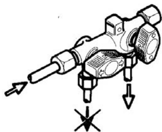
Fig. 74: Posizione di chiusura e di apertura
