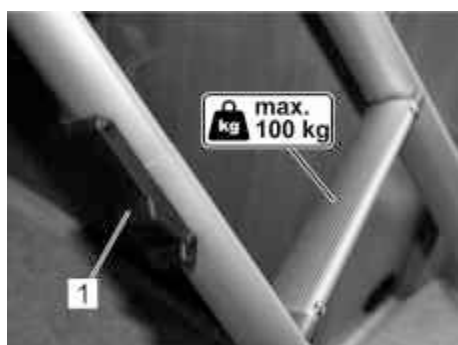
Fig. 186: Meccanismo di bloccaggio (1) della scaletta
