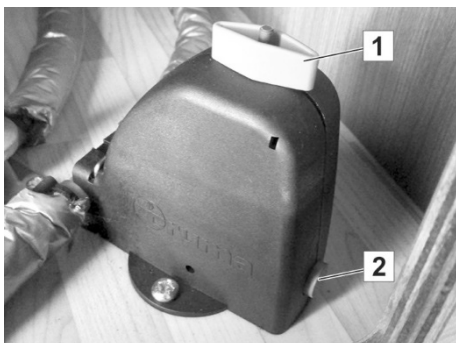
Fig. 104: Valvola di scarico di sicurezza aperta
