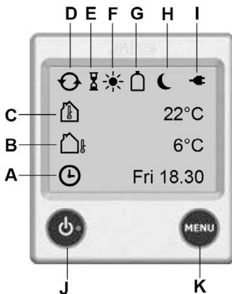
Fig. 81: Elementi di comando
