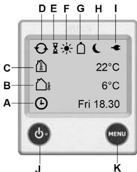
Fig. 155: Elementi di comando
