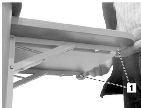
Fig. 206: Allentare l'arresto della mensola ribaltabile
