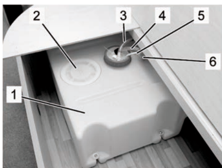
Fig. 89: Serbatoio dell'acqua fresca, esempio
