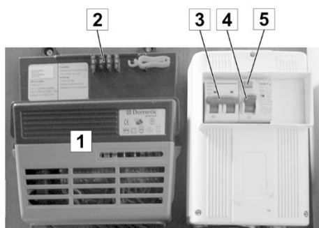
Fig. 57: Convertitore (alimentatore di rete) (1) e interruttori automatici
