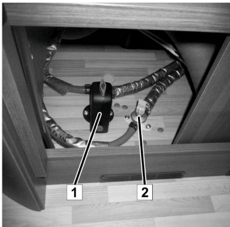
Fig. 103: Valvole di scarico Riscaldamento TRUMA Combi
