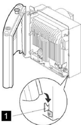
Fig. 127: Rivestimento del riscaldamento aperto
