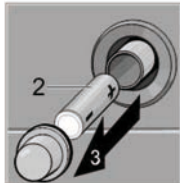
Fig. 214: Sostituzione della batteria con accenditore a batteria (solo se esistente)
