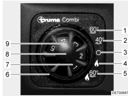
Kuva 80 Säätöyksikkö
