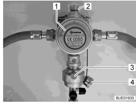
Kuva 60 DuoControl-säätölaiteisto
