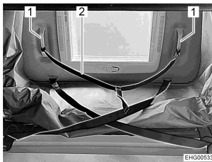
Kuva 57 Apuhihna
