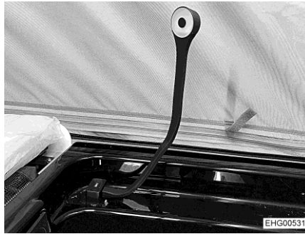
Kuva 55 Joutsenkaulavalaisin, käyttöasento
