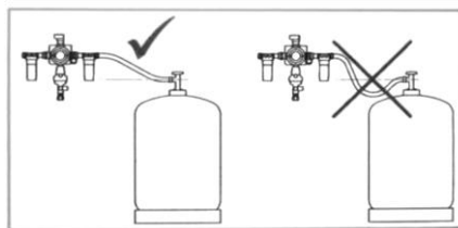
Kuva 62 Kaasupullon kytkeminen oikein
