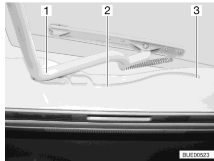
Kuva 23 Ohjaus (Heki-kattoluukku)
