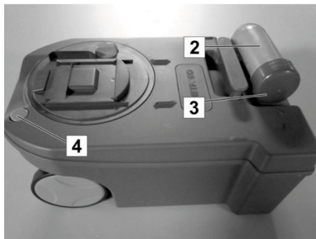
Abb. 140: Fäkalientank entleeren
