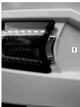
Abb. 157: Heckleuchte abnehmen
