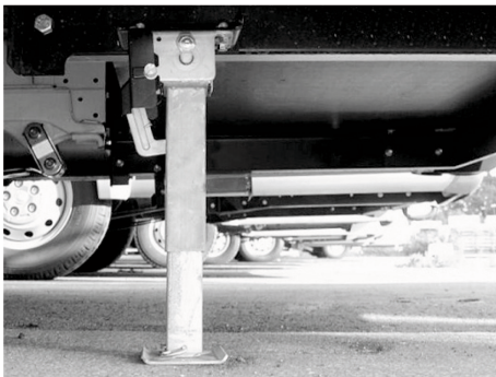
Abb. 15: Heckstütze, ausgefahren
