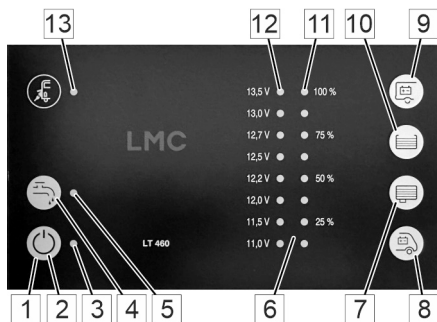
Abb. 56: Bedien- und Kontrollpanel LT 460 A
