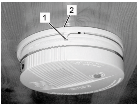
Abb. 162: Gehäuse ansetzen
