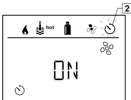
Abb. 108: Anzeige Zeitschaltuhr
