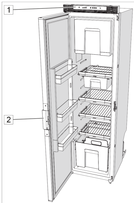
Abb. 148: Kühlschrank Thetford 12 V
