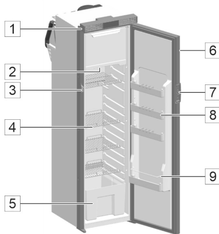
Abb. 146: 12 V-Kompressor-Kühlschrank
