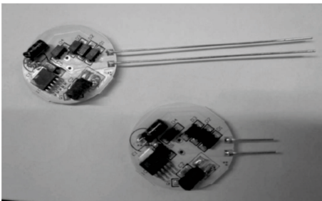
Abb. 151: Kontakte kürzen
