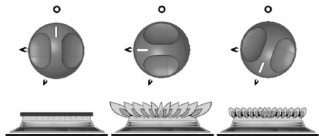
Abb. 143: Stellungen der Bedienelemente: AUS, Hochflamme, Sparflamme
