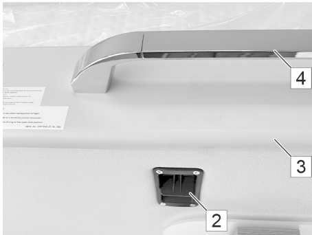
Abb. 128: Arretierung Hubbett (Beispiel)
