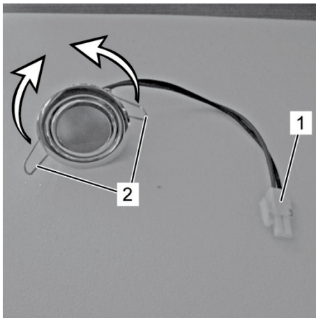
Abb. 155: Übersicht LED
