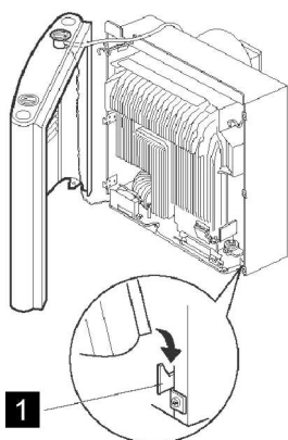
Abb. 134: Heizverkleidung aufgeschwenkt
