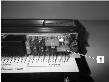
Abb. 75: 12 V-Notbeleuchtung
