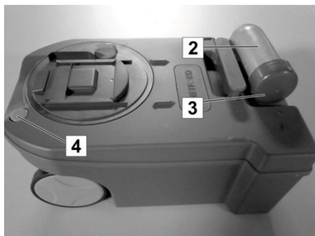
Abb. 162: Fäkalientank entleeren
