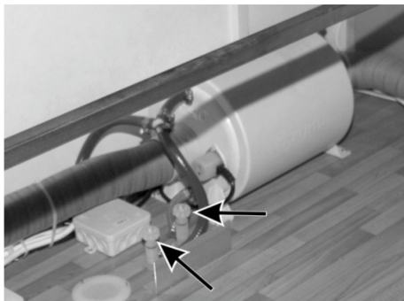
Abb. 103: TRUMA-Therme und Wasserablassventile
