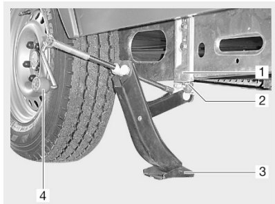
Abb. 176: Wagenheber AL-KO
