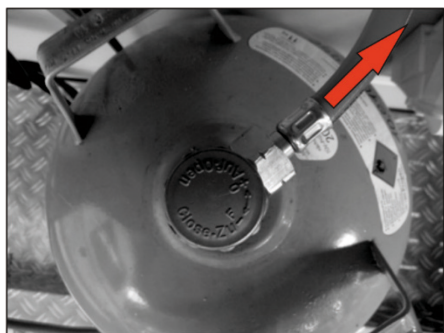
Abb. 88: Ausrichtung Gasflasche
