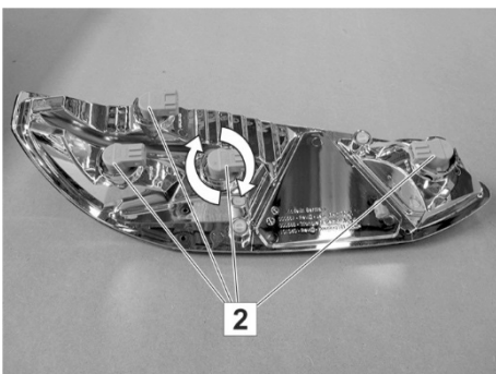
Abb. 180: Heckleuchte (Rückseite)
