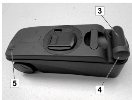
Abb. 159: Fäkalientank entleeren
