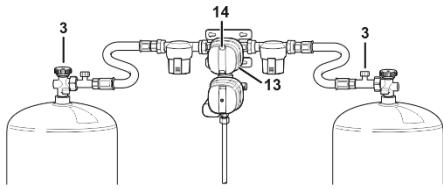
Abb. 115: Gasdruckregler-Set
