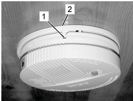
Abb. 121: Gehäuse ansetzen
