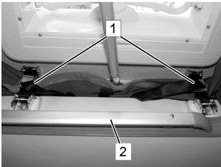
Abb. 151: Aufstelldach aufklappen
