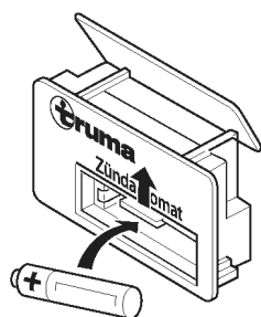
Abb. 135: Batteriewechsel
