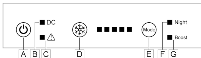
Fig. 171: Elementi di comando del frigorifero a compressore a 12 V
