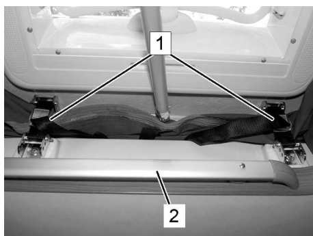
Fig. 151: Aprire il tetto sollevabile ribaltandolo
