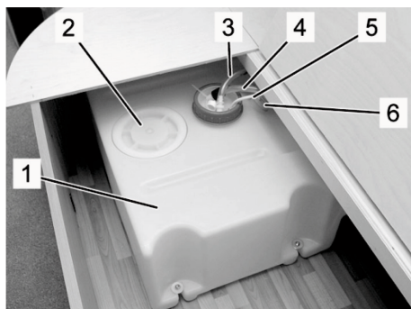
Fig. 98: Serbatoio dell'acqua fresca, esempio
