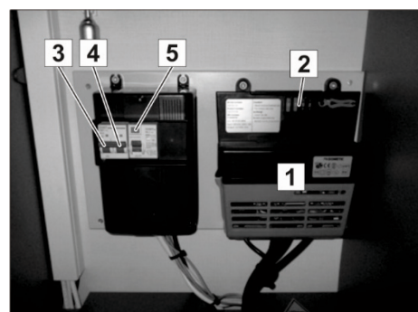
Fig. 74: Convertitore (alimentatore di rete) (1) e interruttori automatici
