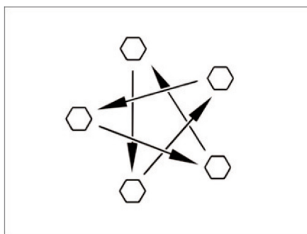
Fig. 172: Serrare in sequenza incrociata i dadi o i bulloni di fissaggio ruota
