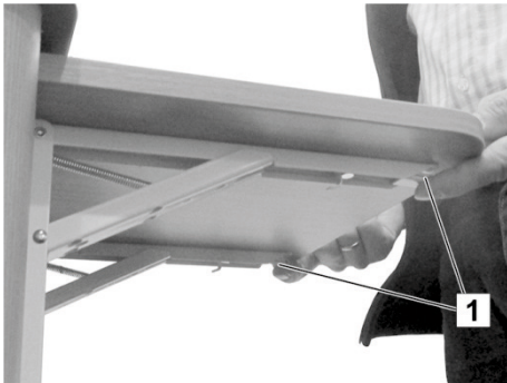
Fig. 167: Allentare l'arresto della mensola ribaltabile
