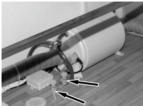
Fig. 139: Valvole di scarico
