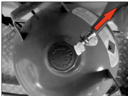
Fig. 88: Allineamento della bombola di gas
