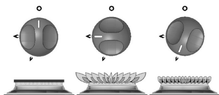
Fig. 165: Posizione degli elementi di comando: OFF, Fiamma alta, Fiamma bassa
