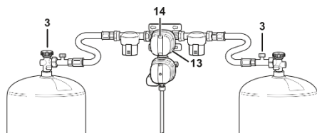
Fig. 118: Set regolatore di pressione del gas
