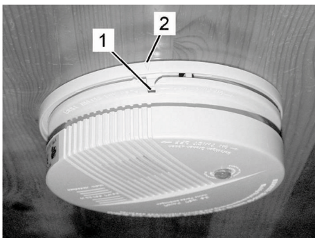
Abb. 171: Gehäuse ansetzen
