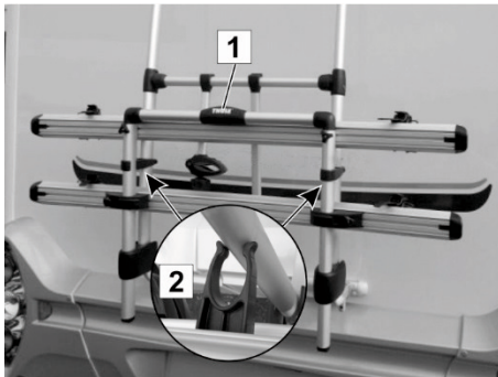
Abb. 27: Fahrradträger ausklappen
