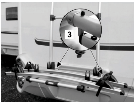
Abb. 28: Arretierungen einrasten
