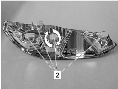
Abb. 167: Heckleuchte (Rückseite)
