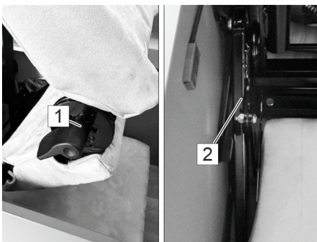
Abb. 16: Klappsitz - Bedienelemente
