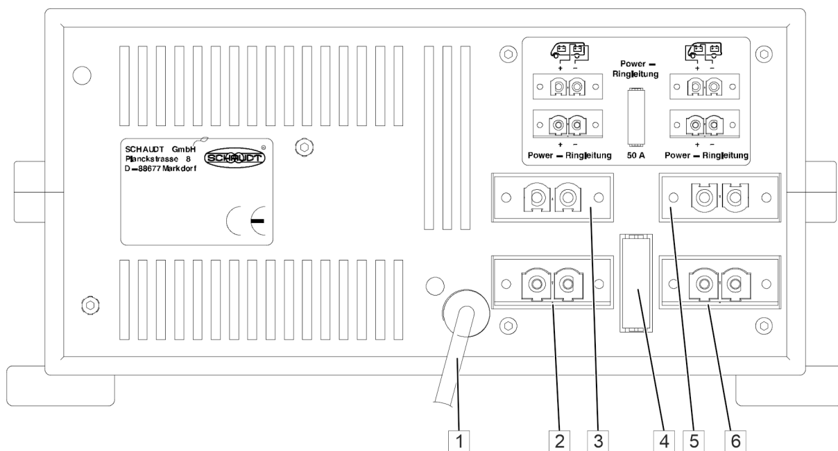
Abb. 5: Anordnung der Sicherungssteckplätze am EBL 400 A (Rückseite)
