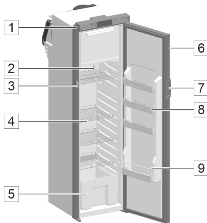
Abb. 157: 12 V-Kompressor-Kühlschrank
