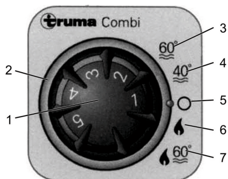
Abb. 77: TRUMA-Bedieneinheit für Heizung und Warmwasserbereitung
