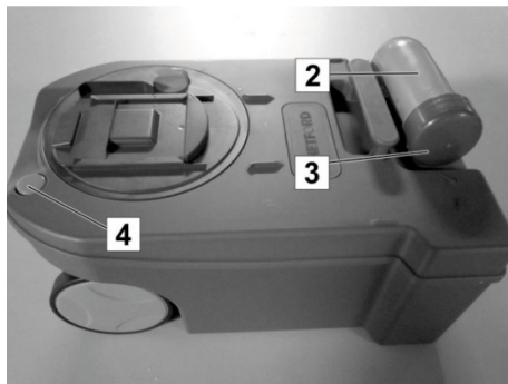
Abb. 151: Fäkalientank entleeren
