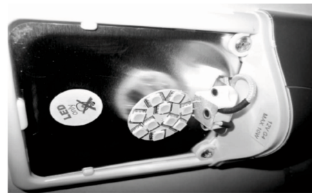
Abb. 161: LED-Leuchtmittel einsetzen
