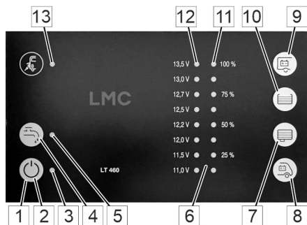
Abb. 61: Bedien- und Kontrollpanel LT 460 A
