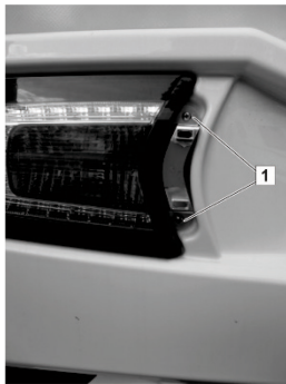
Abb. 168: Heckleuchte anbringen
