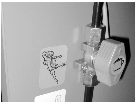
Abb. 72: Schnellschlussventile
