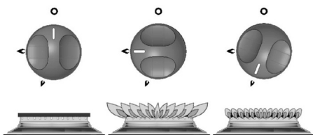
Abb. 154: Stellungen der Bedienelemente: AUS, Hochflamme, Sparflamme
