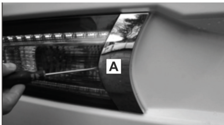
Abb. 165: Heckleuchte
