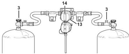
Abb. 98: Gasdruckregler-Set
