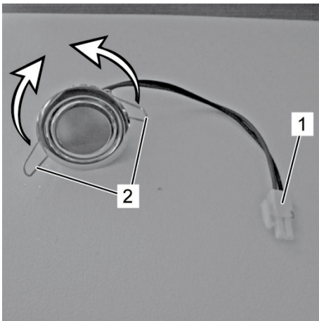
Abb. 164: Übersicht LED
