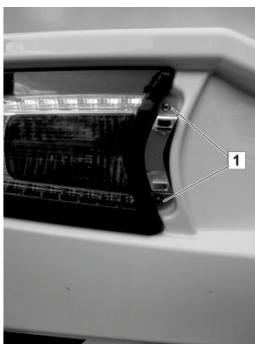
Abb. 166: Heckleuchte abnehmen
