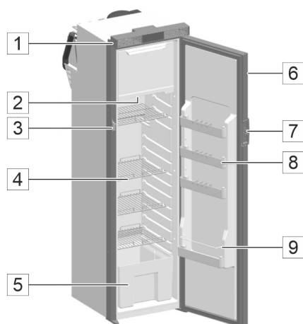
Fig. 157 : Réfrigérateur à compression 12 V
