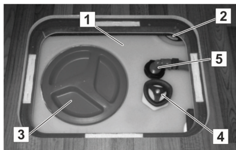
Fig. 89 : Disposition sous le plancher
