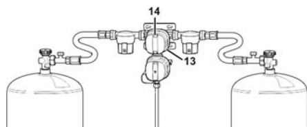
Fig. 118 : Kit détendeur
