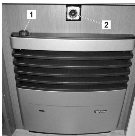
Fig. 130: Chauffage TRUMA
