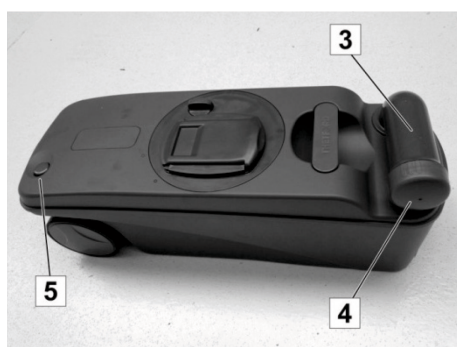
Fig. 159 : Vidange de la cassette WC
